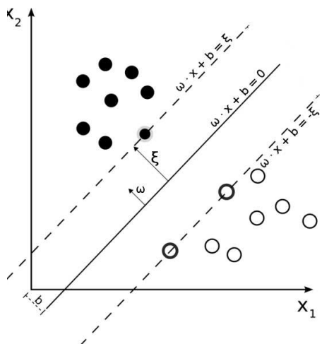
Figura 2: Representación gráfica de la función de clasificación de SVM.
